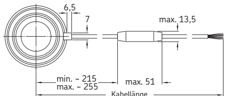
008A (mit freiem Kabelende)
