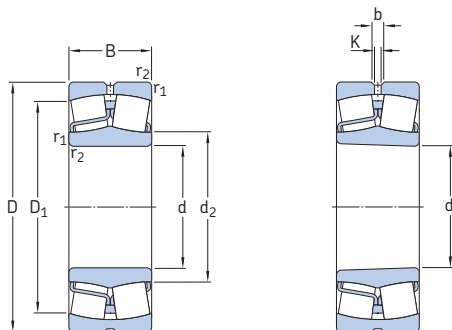
Zylindrische Bohrung
