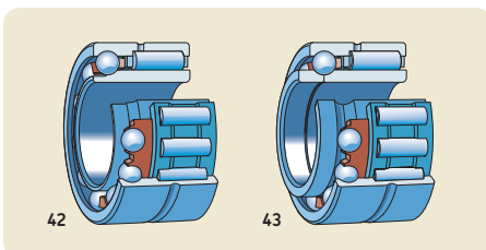
Kombinierte Nadellager Nadel-/Schräggugellager einseitig wirkend (42) zweiseitig wirkend (43)
