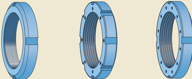
KM(L) / HM.. T / AN / N (Größe \leq 44 )
