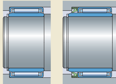
Mit Standard-Innenring
