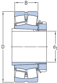
Lager auf Spannhülse der Grundausführung
