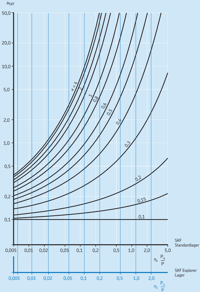
Lebensdauerbeiwert a_{SKF} für Radial-Kugellager
