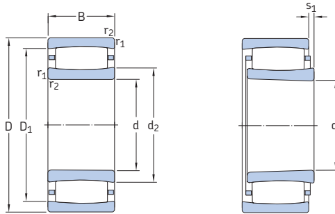
Zylindrische Bohrung
