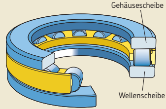
Einreihiges Lager, Reihen 811 und 812
