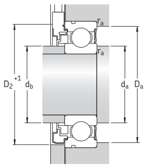
Bohrungsdurchmesser des Enddeckels \geq D_2 + 1 mm
