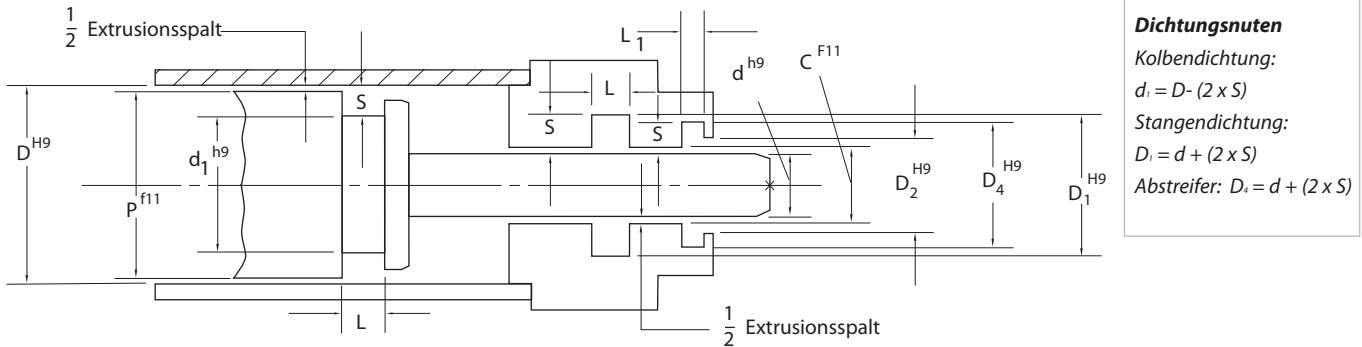
Abb. 1 Die Beispiele unten illustrieren, wie Passungen und Toleranzen zur Bemessung einer oder mehrerer Komponenten des in Abbildung 1 für metrische und US-Größen gezeigten Zylinders angewendet werden können.
